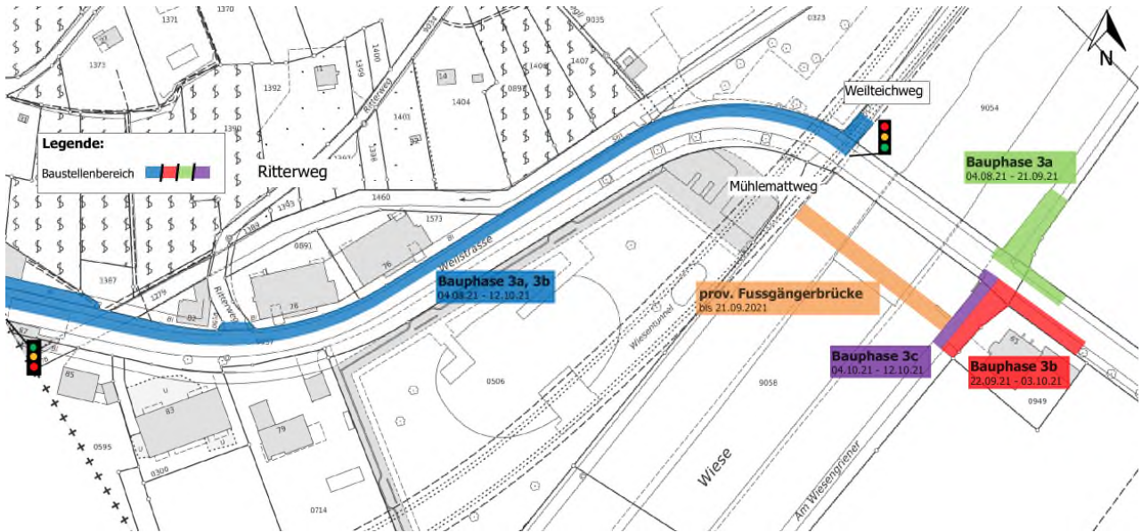
Abb. 3: Bauphasen 3a bis 3c vom 04.08.2021 bis 12.10.2021
