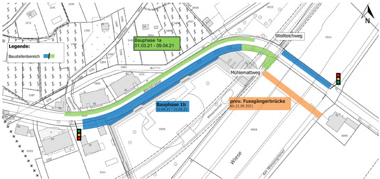
Abb. 1: Bauphasen 1a und 1b vom 8.03. bis 21.05.2021
